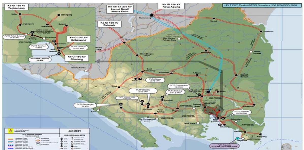
Gambar 2. 30 Peta Sistem Tenaga Listrik Provinsi Lampung
